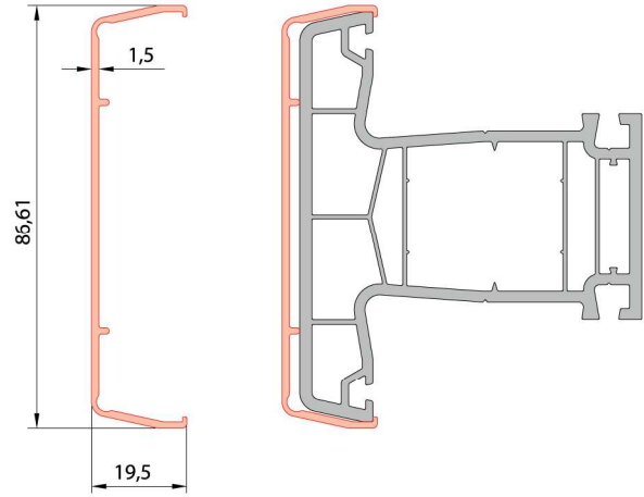
Alüminyum Giydirm Orta Kayıt Profili
