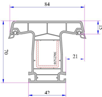
Orta Kayıt Profili Kod: P.A.750.3000.600.0.BC.01
