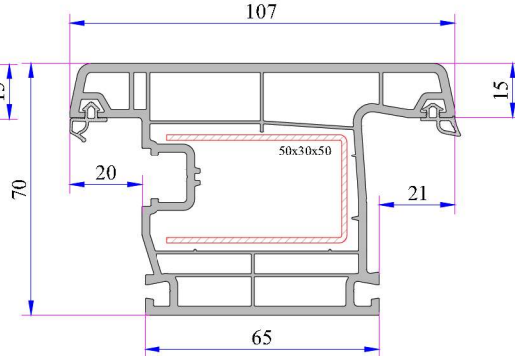
Dışa Açılım Kapı Kanat Profili Kod: P.A.750.2101.600.0.BC.01
