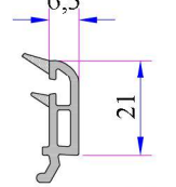
42 mm Contalı Üçlü Cam Çıtası Kod: P.A.532.4500.600.0.HC
