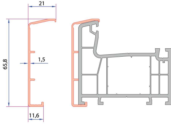
Alm. Giydirm Normal Kasa Profili
