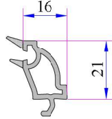
32 mm Dekoratif Contalı Üçlü Cam Çıtası Kod: P.A.101.4202.600.0.HC
