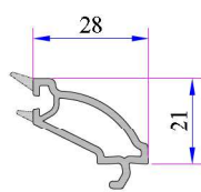
20 mm Dekoratif Contalı Çift Cam Çıtası Kod: P.A.750.4102.600.0.HC
