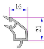
32 mm Contalı Üçlü Cam Çıtası Kod: P.A.750.4500.600.0.HC
