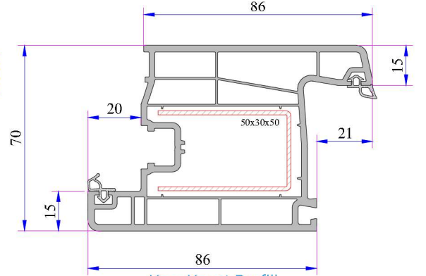
Kapı Kanat Profili Kod: P.A.750.2100.600.0.BC.01
