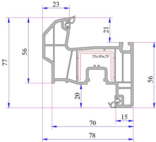
Damlalıklı Kanat Profili (6 Odacıklı) Kod: P.A.750.2205.600.0.BC.01
