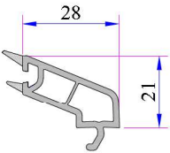
20 mm Contalı Çift Cam Çıtası Kod: P.A.750.4100.600.0.HC
