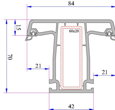
Süper Statik Orta Kayıt Profili Kod: P.A.750.3009.600.0.BC.01
