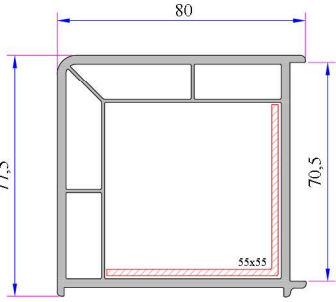
90° Köşe Profili Kod: P.A.070.5100.600.0.00.19
