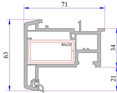
Statik Hareketli Orta Kayıt Profili (Tırnaklı) Kod: P.A.750.3101.600.0.BC.19
