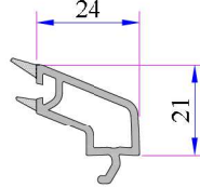
24 mm Contalı Çift Cam Çıtası Kod: P.A.750.4200.600.0.HC
