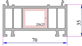
Kasa Yükseltme Profili 35mm Kod: P.A.070.5300.600.0.00.19
