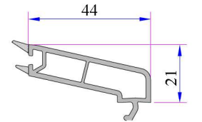
4-6 mm Contalı Tek Cam Çıtası Kod: P.A.750.4000.600.0.HC
