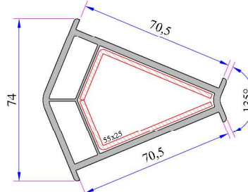
135° Köşe Profili Kod: P.A.070.5102.600.0.00.19
