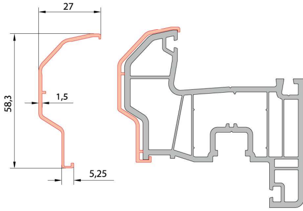
Alüminyum Giydirm Damlalıklı Kanat Profili
