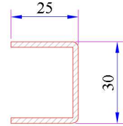
Kanat-Damlalık Kanat Profili Destek Sacı Kod: 34022-12025
