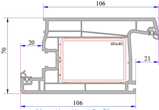
Süper Kapı Kanat Profili Kod: P.A.750.2103.600.0.BC.01
