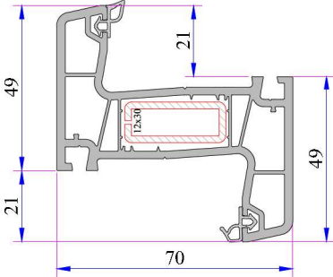
Dışa Açılım Orta Kayıt Profili Kod: P.A.750.3005.600.0.BC.0
