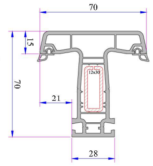
Eko Orta Kayıt Profili Kod: P.A.750.3006.600.0.BC.01
