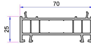
Kasa Yükseltme Profili 25 mm Kod: 070.5306
