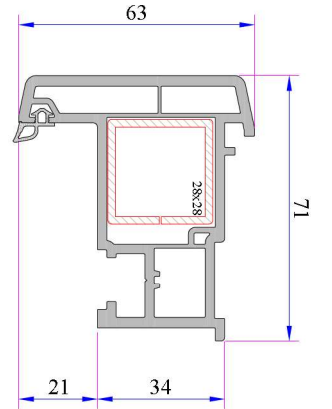
Hareketli Orta Kayıt Profili Kod: P.A.750.3100.600.0.BC.19
