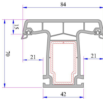
Statik Orta Kayıt Profili Kod: P.A.750.3007.600.0.BC.01
