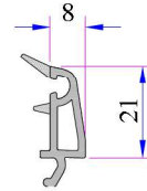
40 mm Contalı Üçlü Cam Çıtası Kod: P.A.532.4400.600.0.HC
