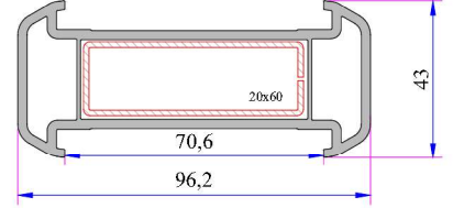
Kalın Bağ Profili Kod: P.A.070.5000.600.0.00.19
