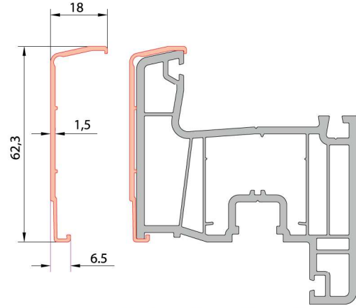
Alüminyum Giydirm Normal Kanat Profili
