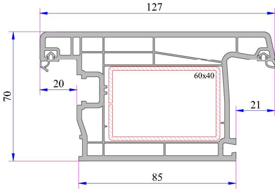
Dışa Açılım Süper Kapı Kanat Profili Kod: P.A.752.2104.600.0.BC.01
