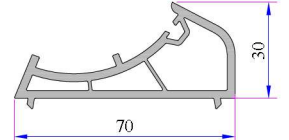
Açılı Dönüş Adaptör Profili Kod: P.A.070.5104.600.0.00.19
