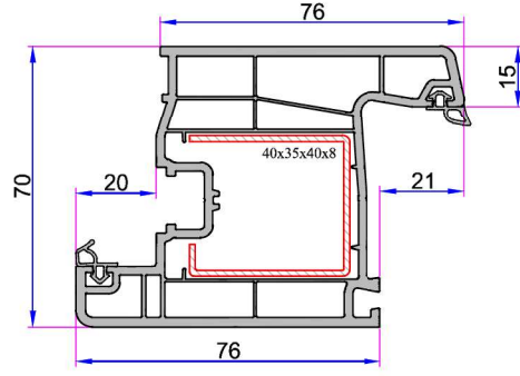
Dar Kapı Kanat Profili Kod: P.A.750.2111.600.0.BC.01
