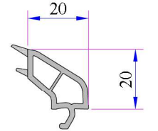
28 mm Contalı Çift Cam Çıtası Kod: P.A.101.4100.600.0.HC
