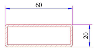
Statik Orta Kayıt Profili Destek Sacı Kod: 34022-12106
