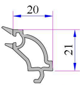
28 mm Dekoratif Contalı Çift Cam Çıtası Kod: P.A.101.4102.600.0.HC
