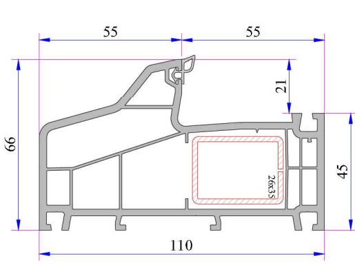
W 790 Kasa Profili
