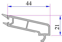
4-6 mm Contalı Tek Cam Çıtası Kod: P.A.750.4000.600.0.HC
