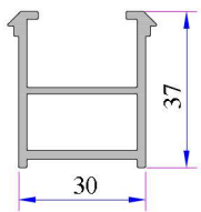
Kasa Montaj Profili Kod: P.A.060.5301.600.0.00.19
