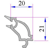
28 mm Dekoratif Contalı Çift Cam Çıtası Kod: P.A.101.4102.600.0.HC
