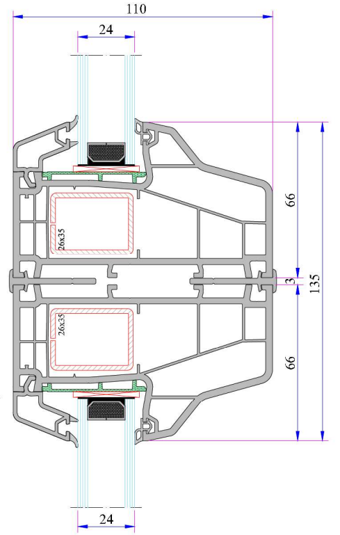
İnce Bağ Profili Montajı
