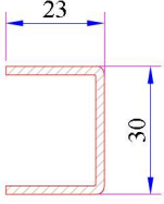
24 Aks Kanat Profili Destek Sacı Kod: 34022-12030
