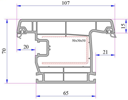
Dışa Açılım Kapı Kanat Profili Kod: P.A.750.2101.600.0.BC.01
