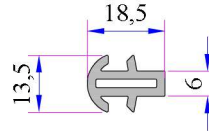
Dışa Açılım Süper Kapı Kanat Profili Kod: P.A.752.2104.600.0.BC.01
