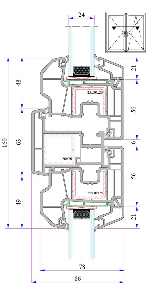
Kanat - Hareketli Orta Kayıt Montajı
