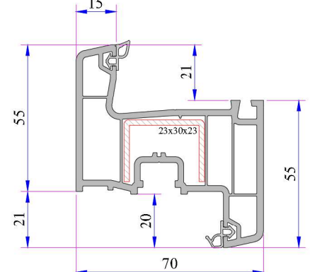
24 Aks Kanat Profili
