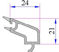
24 mm Contalı Çift Cam Çıtası Kod: P.A.750.4200.600.0.HC
