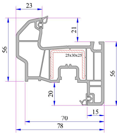
Damlalıklı Kanat Profili
