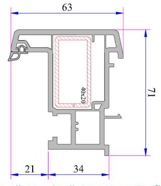
Statik Hareketli Orta Kayıt Profili (Tırnaklı) Kod: P.A.750.3101.600.0.BC.19
