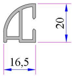
Damlalık Profili Kod: P.A.900.6307.600
