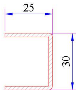
Kasa - Damlalıklı Kanat Profili Destek Sacı Kod: 34022-12025
