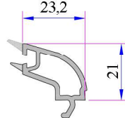
24 mm Dekoratif Contalı Çift Cam Çıtası Kod: P.A.750.4204.600.0.HC
