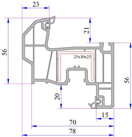
Damlalıklı Kanat Profili (6 Odacıklı)
