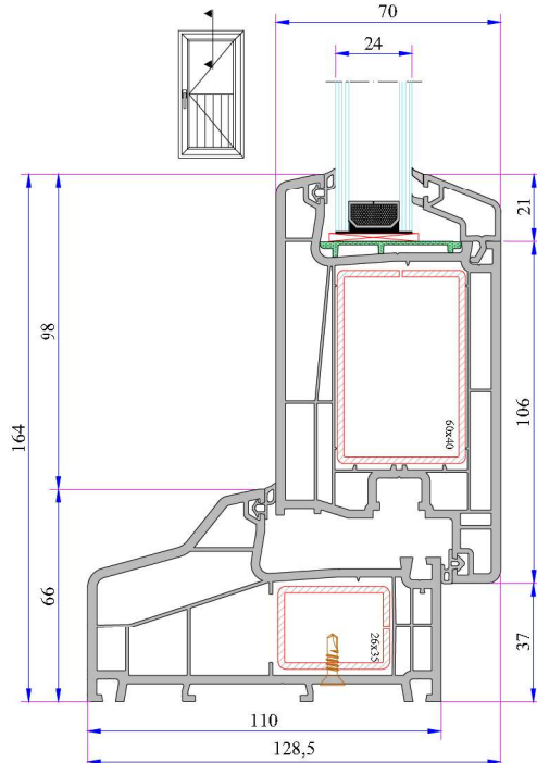
Kasa - Süper Kapı Kanat Montajı
