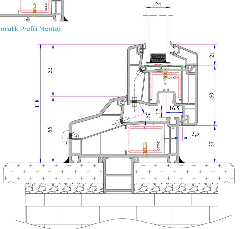
Kasa Montaj Profili Kullanım Detayı
