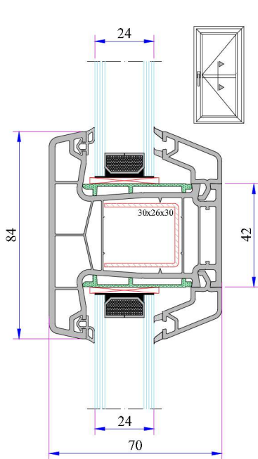
Kapı İçi Orta Kayıt Montajı
