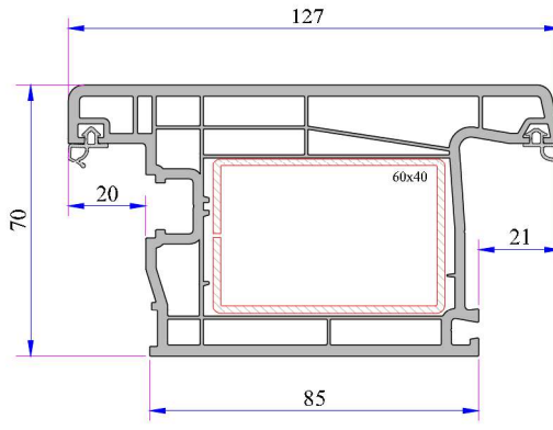
Dışa Açılım Süper Kapı Kanat Profili Kod: P.A.752.2104.600.0.BC.01
