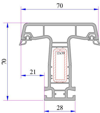
Eko Orta Kayıt Profili
