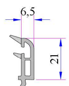
42 mm Contalı Üçlü Cam Çıtası Kod: P.A.532.4500.600.0.HC
