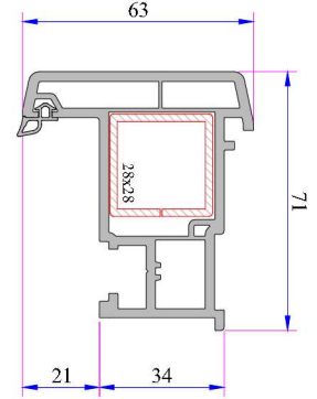
Hareketli Orta Kayıt Profili Kod: P.A.750.3100.600.0.BC.19
