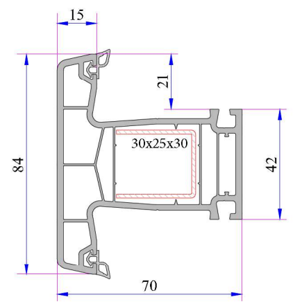
Kapı İçi Orta Kayıt Profili
