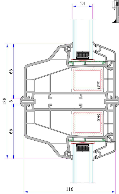
Kısa Bağ Profili Montajı
