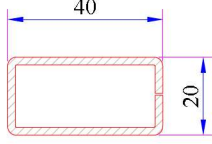
Statik hareketli Orta Kayıt Profili Destek Sacı Kod: 34022-12114
