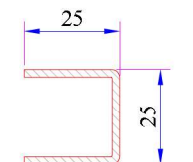
Dışa Açılım Kanat Profili Destek Sacı Kod: 34022-12003
