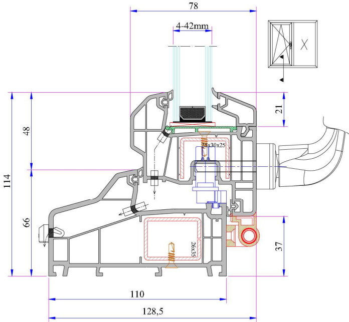
Kasa - Kanat Montajı
