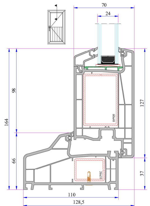
Kasa - Dışa Açılım Süper Kapı Kanat Montajı
