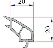
28 mm Contalı Çift Cam Çıtası Kod: P.A.101.4100.600.0.HC
