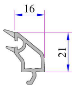
32 mm Contalı Üçlü Cam Çıtası Kod: P.A.750.4500.600.0.HC
