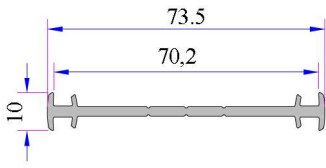
İnce Bağ Profili Kod: P.A.070.5001.600
