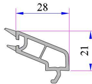
20 mm Contalı Çift Cam Çıtası Kod: P.A.750.4100.600.0.HC
