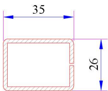
Kasa - Orta Kayıt Destek Sacı Kod: 34022-12116
