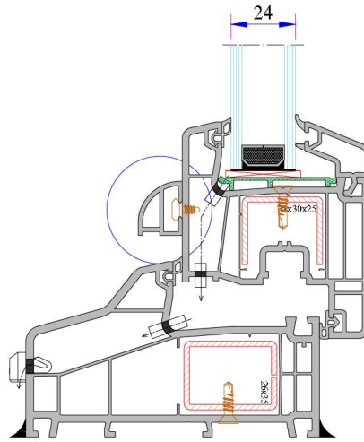
Damlalık Profili Montajı
