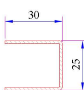
Kapı İçi Orta Kayıt Profili Destek Sacı Kod: 34022-12004
