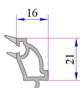
32 mm Dekoratif Contalı Üçlü Cam Çıtası Kod: P.A.101.4202.600.0.HC
