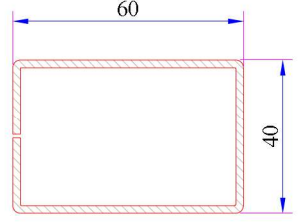
Süper Kapı Kanat - Dışa Açılım Süper Kapı Kanat Profili Destek Sacı Kod: 34022-12110
