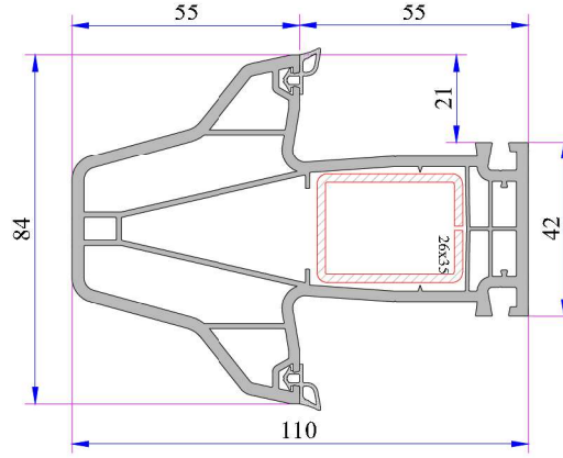
W 790 Orta Kayıt Profili
