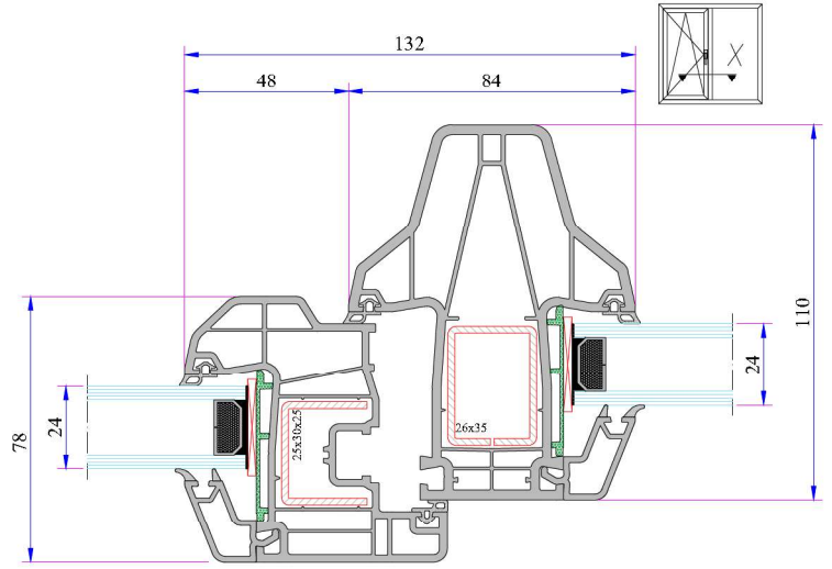
Orta Kayıt - Damlalıklı Kanat Montajı
