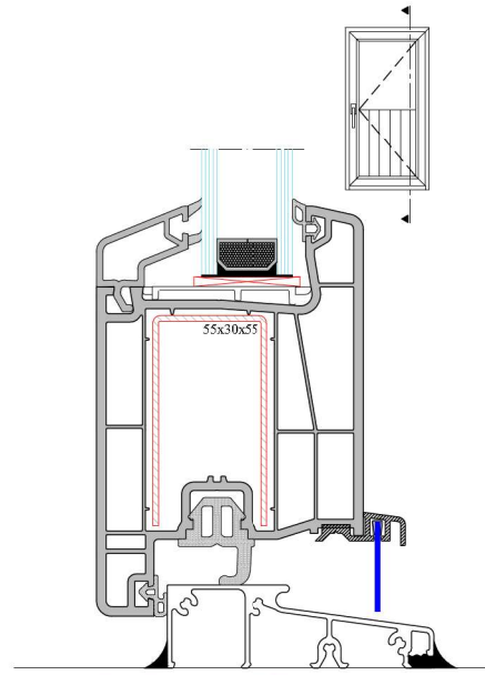
Alüminyum Eşikli Kasa - Kapı Kanat Montajı
