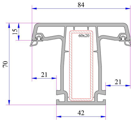
Statik Orta Kayıt Profili
