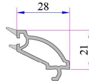
20 mm Dekoratif Contalı Çift Cam Çıtası Kod: P.A.750.4102.600.0.HC
