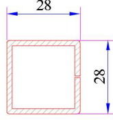
Hareketli Orta Kayıt Profili Destek Sacı Kod: 34022-12113
