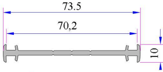
İnce Bağ Profili
