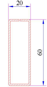
Kalın Bağ Profili Destek Sacı Kod: 34022-12106
