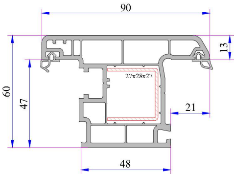
Dışa Açılım Kanat Profili (9 Aks)
