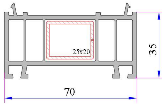
Kasa Yükseltme Profili 35mm
