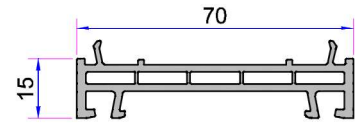
Kasa Yükseltme Profili 15 mm
