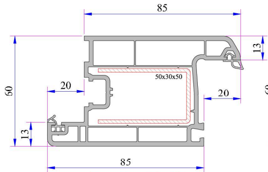
Kapı Kanat Profili
