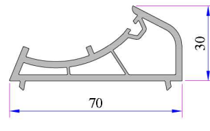
Açılı Dönüş Adaptör Profili
