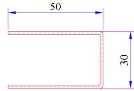
Kapı Kanat - Dışa Açılım Kapı Kanat Profili Destek Sacı Kod: 34022-12013
