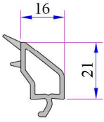
24 mm Contalı Çift Cam Çıtası
