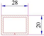
Hareketli Orta Kayıt Profili Destek Sacı Kod: 34022-12118
