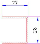
Dışa Açılım Kanat Profili Destek Sacı (9 Aks) Kod: 34022-12020
