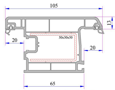
Dışa Açılım Kapı Kanat Profili
