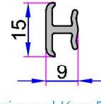
Universal Kısa Bağ Profili
