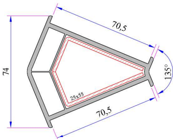
135° Köşe Profili
