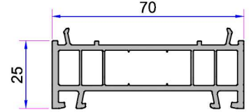
Kasa Yükseltme Profili 25 mm
