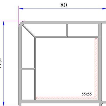
90° Köşe Profili
