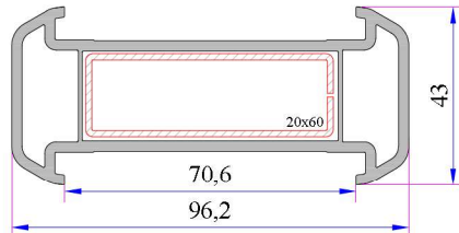
Kalın Bağ Profili
