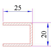
Pervazlı Kasa Profili Destek Sacı Kod: 34022-12021
