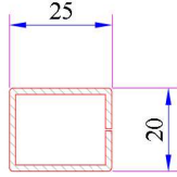
35mm Kasa Yükseltme Profili Destek Sacı Kod: 34022-12104
