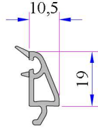
30 mm Contalı Üçlü Cam Çıtası
