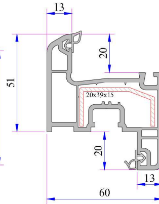
Dar Kanat Profili
