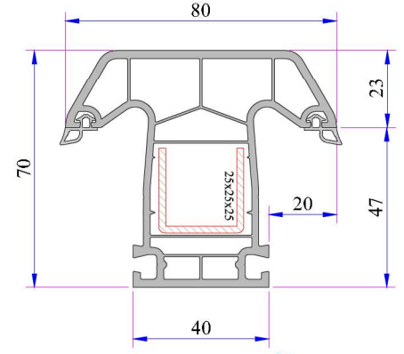
Orta Kayıt Profili
