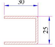
Kapı İçi Orta Kayıt Profili Destek Sacı Kod: 34022-12004
