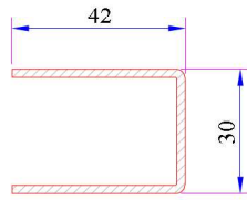
Eko Kapı Kanat - Dışa Açılım Eko Kapı Kanat Profili Destek Sacı Kod: 34022-12023
