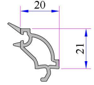
20 mm Dekoratif Contalı Çift Cam Çıtası
