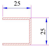
332 Kanat Profili Destek Sacı Kod: 34022-12003
