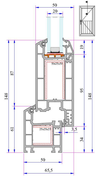
332 Kasa - Kapı Kanat Montajı
