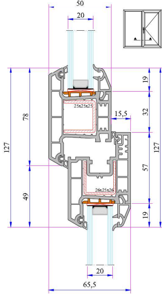
332 Orta Kayıt - Kanat Montajı
