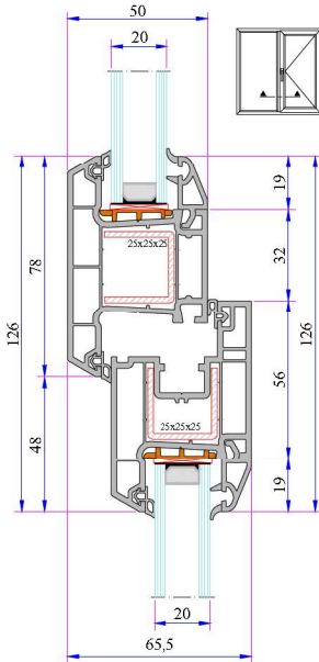
330 Orta Kayıt - Kanat Montajı
