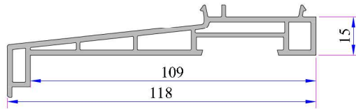
Kasa Altı 110mm Takma Denizlik
