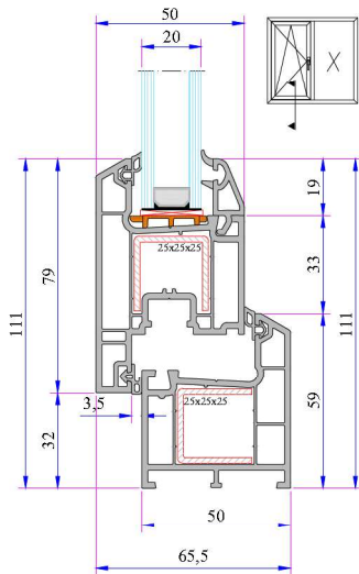
330 Kasa - Dışa Açılım Kanat Profili
