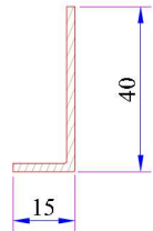
135° Köşe Dönüş Profili Destek Sacı Kod: 34022-12301
