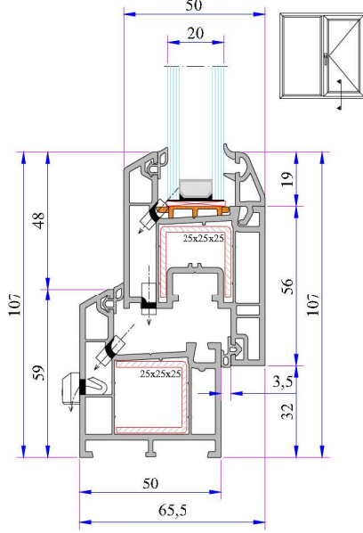
330 Kasa - Kanat Montajı
