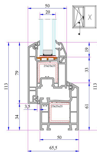
332 Kasa - Dışa Açılım Kanat Montajı
