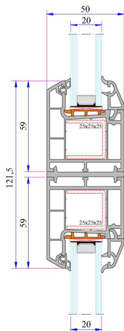
330 Kasa - İnce Bağ Profili Montajı
