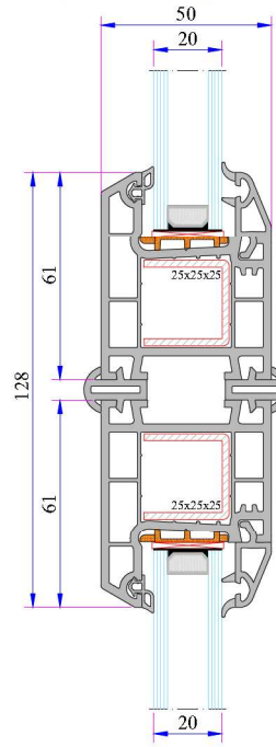
332 Kasa - Kısa Bağ Profili Montajı
