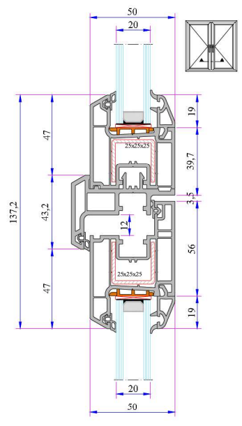
330 Kanat - Hareketli Orta Kayıt Montajı
