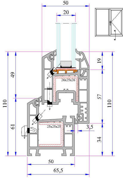
332 Kasa - Kanat Montajı
