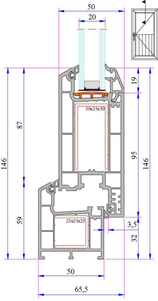
330 Kasa - Kapı Kanat Montajı
