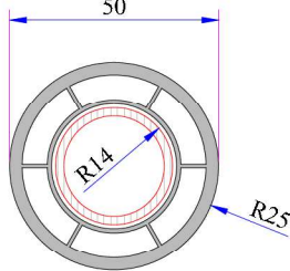
Ø50 Açılı Dönüş Borusu Kod: P.A.050.5106.600
