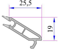
4 mm Contalı Tek Cam Çitası Kod: P.A.332.4000.600.0.HC
