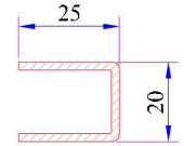
330 Pervazlı Kasa Profili Destek Sacı Kod: 34022-12021
