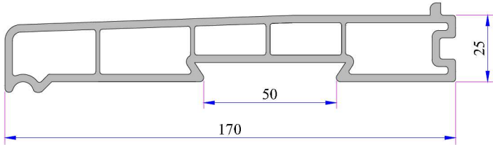
Denizlik Profili 170mm Kod: P.A.099.5513.600.0.00.19
