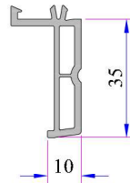
Kasa Altı Klips Pervaz Profili (35mm) Kod: P.A.099.5523.600
