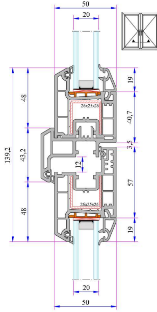
332 Kanat - Hareketli Orta Kayıt Montajı
