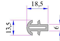
Kısa Bağ Profili Kod: P.A.099.5003.600
