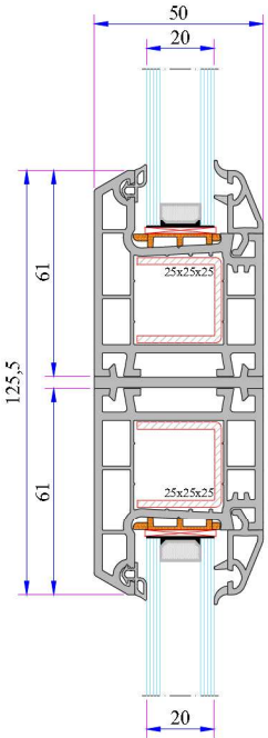
332 Kasa - İnce Bağ Profili Montajı
