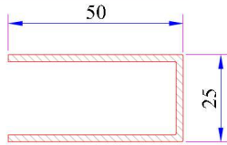
332 Kapı Kanat Profili Destek Sacı Kod: 34022-12012
