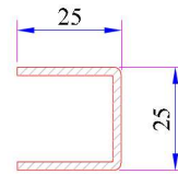
330 Kasa - Kanat - Orta Kayıt - Dışa Açılım Kanat Profili Destek Sacı Kod: 34022-12003
