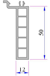
Kasa Altı Klips Pervaz Profili (50mm) Kod: P.A.099.5524.600
