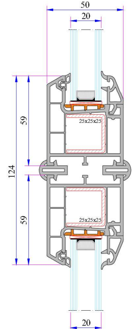
330 Kasa - Kısa Bağ Profili Montajı
