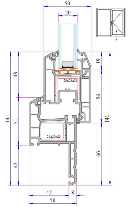
330 Pervazlı Kasa - Kanat Montajı
