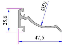
Alm. Açılı Köşe Dönüş Adaptörü (Yeni Yapılacak)
