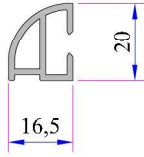
Damlalık Profili Kod: P.A.900.6307.600
