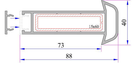
Üniversal Kalın Bağ Profili Kod: P.A.058.5000.600.0.00.19
