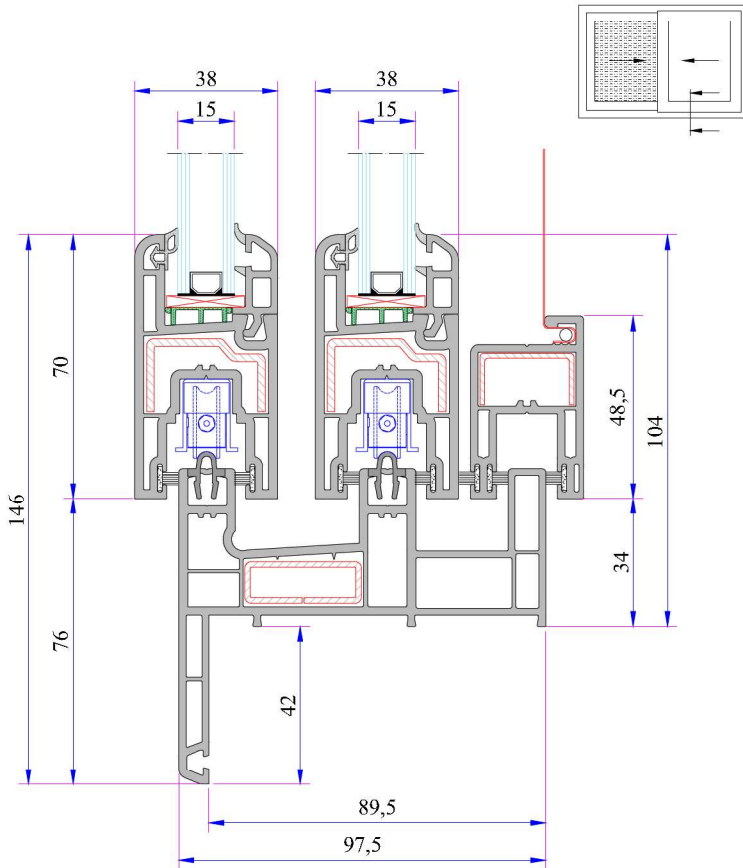
Sürme Pervazlı Sineklik Kasa - Sürme Kanat Montaj Detayı
