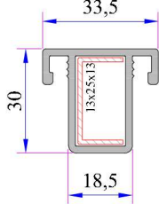
Sineklik Orta Kayıt Profili Kod: P.A.242.3200.600.0.00.03
