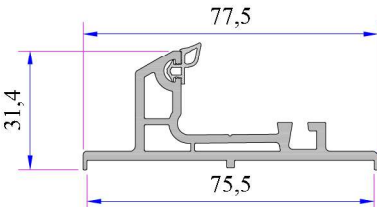
Çift Ray Adaptör Profili Kod: P.A.232.5800.600.0.BC.19
