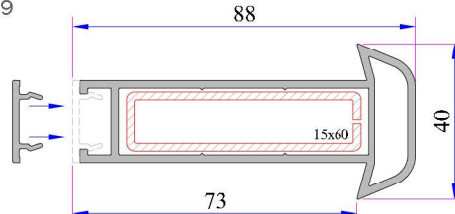
Ünlversal Kalın Bağ Profili Kod: P.A.058.5000.600.0.19
