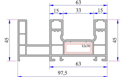
Sürme Sineklik Raylı Kasa Profili Kod: P.A.222.1113.600.0.00.01
