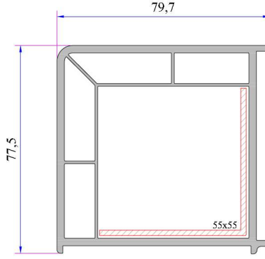
90° Köşe Dönüş Profili Kod: P.A.070.5100.600.0.00.19
