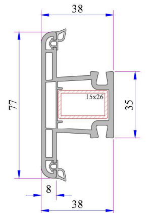
Kanat İçi Orta Kayıt Profili Kod: P.A.222.3201.600.0.BC.01
