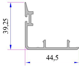
222 Sürme Alın Kapama Kod: P.A.222.5708.600
