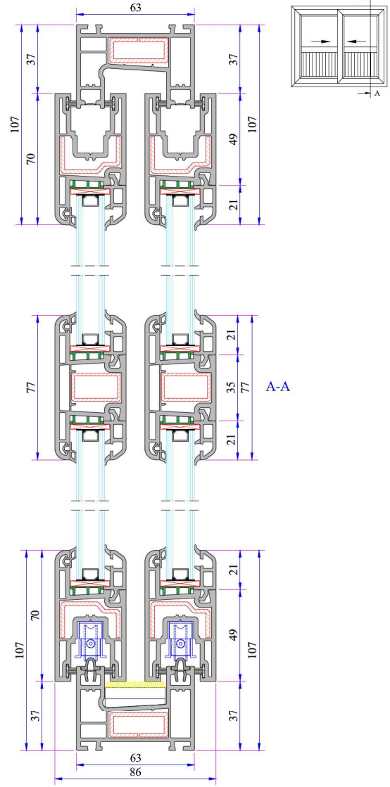
Kanat İçi Orta Kayıt Montaj Detay
