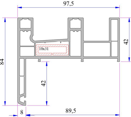
Sürme Pervazlı Sineklik Kasa Profili Kod: P.A.222.1109.600.0.00.01
