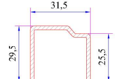
Süper Sürme Kanat Profili Destek Sacı Kod: 34022-15027
