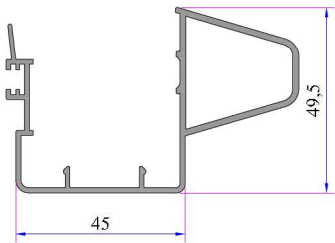
Alm. Kanat Kapama Griyaj Profili (Yeni Yapılacak)
