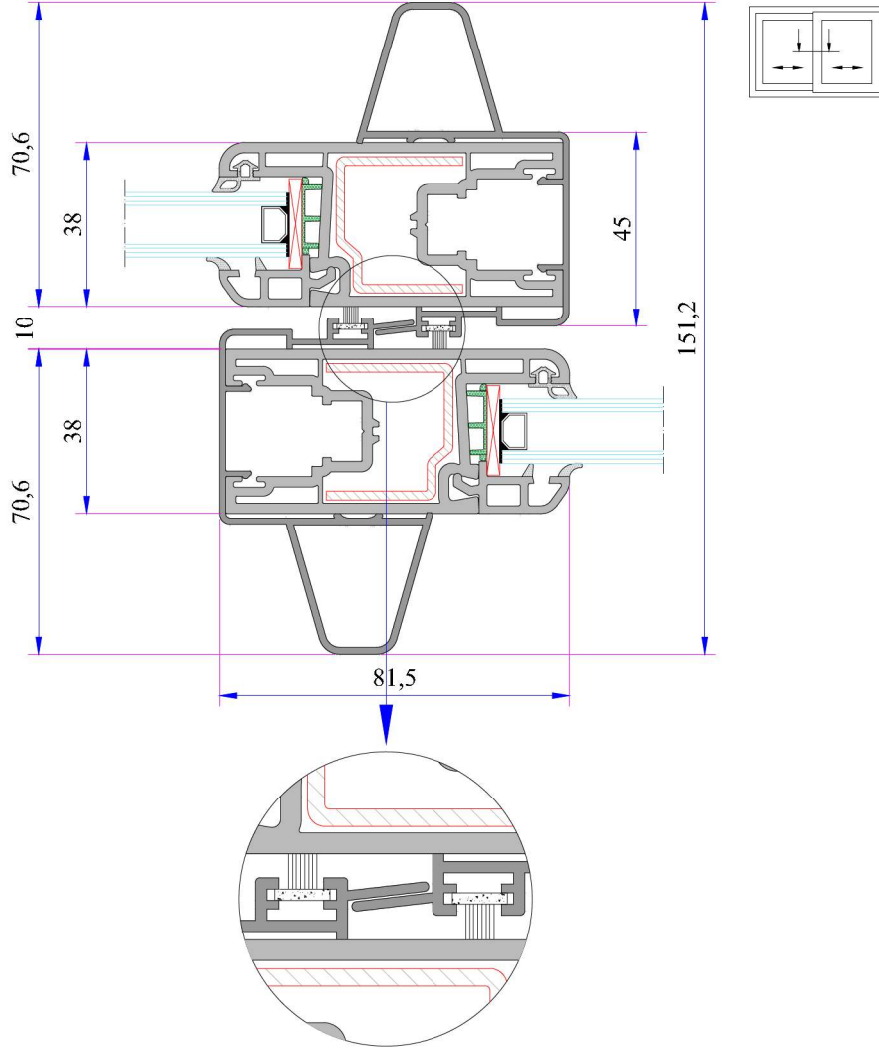
Alm. Çift Ray Adaptörü Montaj Detayı
