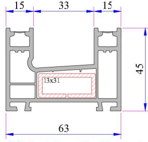
Çift Raylı Kasa Profili (Yeni) Kod: P.A.222.1111.600.0.00.01
