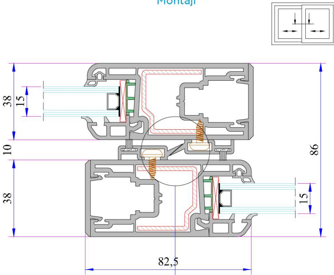
Süper Sürme Kanat Alm. Arka Kapama Montajı
