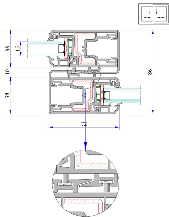
Sürme Kanat Arka Kapama Montajı
