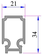
Alm. Çift Ray Adaptörü Kod: 16011.601.5.1.1.9016
