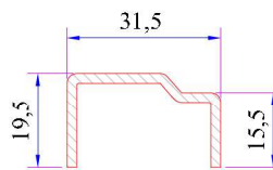
Sürme Kanat Profili Destek Sacı Kod: 34022-15026
