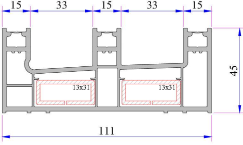
Üç Raylı Kasa Profili (Yeni) Kod: P.A.222.1112.600.0.00.01
