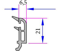
Çift Cam Çıtası 17mm Kod: P.A.532.4500.600.0.HC
