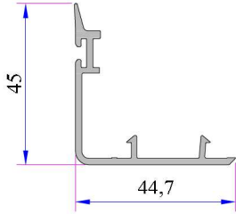
PVC Süper Kanat Arka Kapama Kod: P.A.222.5700.600.0.00.19
