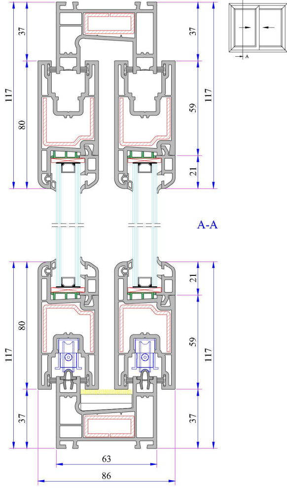
Çift Raylı Kasa İkili Kanat Montaj Detayı
