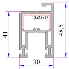
Sürme Sineklik Kanat Profili Kod: P.A.242.2305.600.0.00.03
