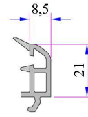
Çift Cam Çıtası 15mm Kod: P.A.532.4400.600.0.HC
