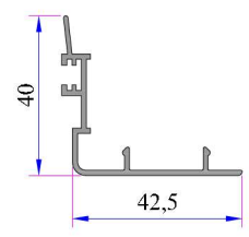
Alm. Kanat Arka Kapama Kod: 16031.601.5.1.1.9016
