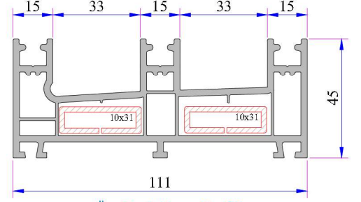
Üç Raylı Kasa Profili Kod: P.A.222.1103.600.0.00.01
