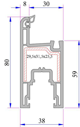
Süper Sürme Kanat Profili Kod: P.A.222.2304.600.0.BC.01
