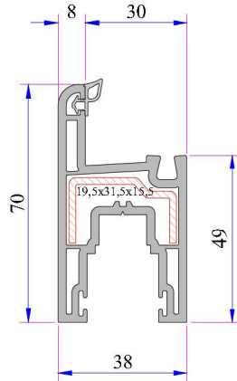
Sürme Kanat Profili Kod: P.A.222.2300.600.0.BC.01
