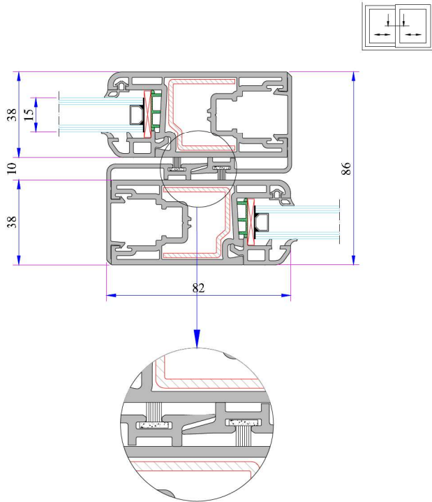
Süper Sürme Kanat Arka Kapama Montajı
