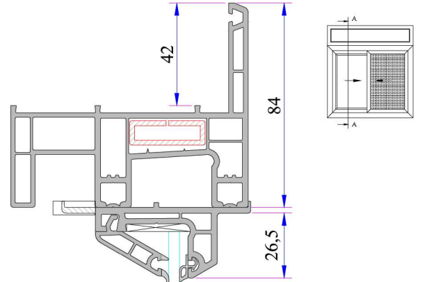
Çift Ray Adaptör Profili Montajı
