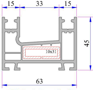
Çift Raylı Kasa Profili Kod: P.A.222.1100.600.0.00.01
