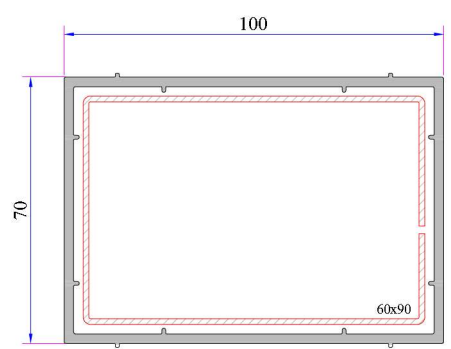
Kutu Profili 70x100mm Kod: P.A.070.5202.600.0.00.19
