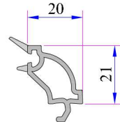
Tek Cam Çıtası 4-6mm Kod: P.A.101.4002.600.0.HC
