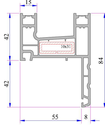
Çift Raylı Pervazlı Kasa Profili Kod: P.A.222.1107.600.0.00.01
