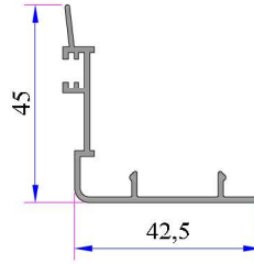
Alm. Süper Kanat Arka Kapama Kod: 16032.601.5.1.1.9016
