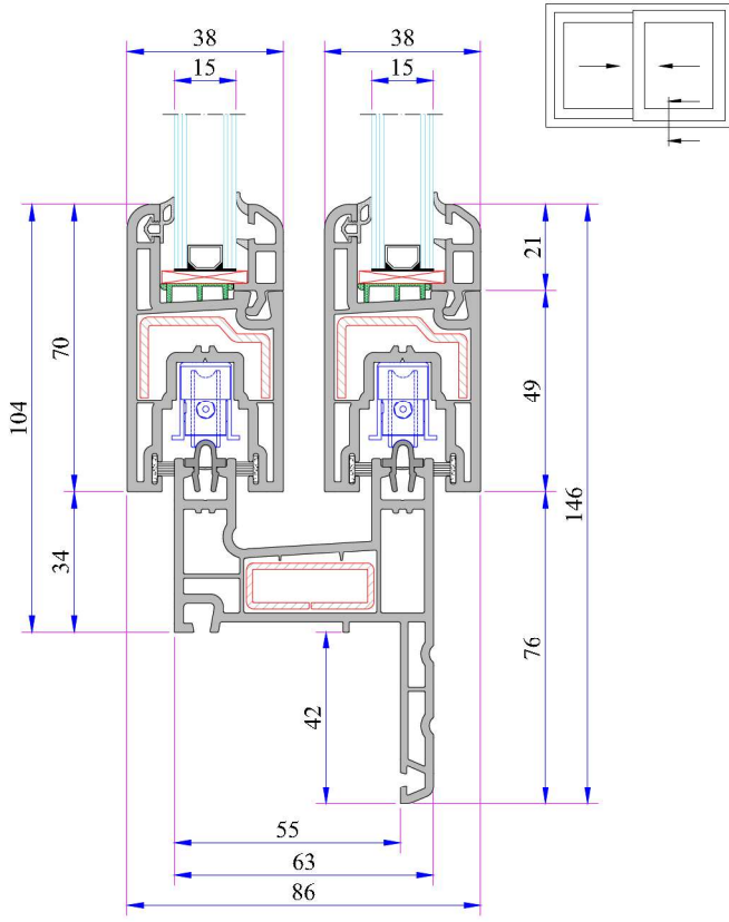
Pervazlı Çift Raylı Kasa - Sürme Kanat Montaj Detayı
